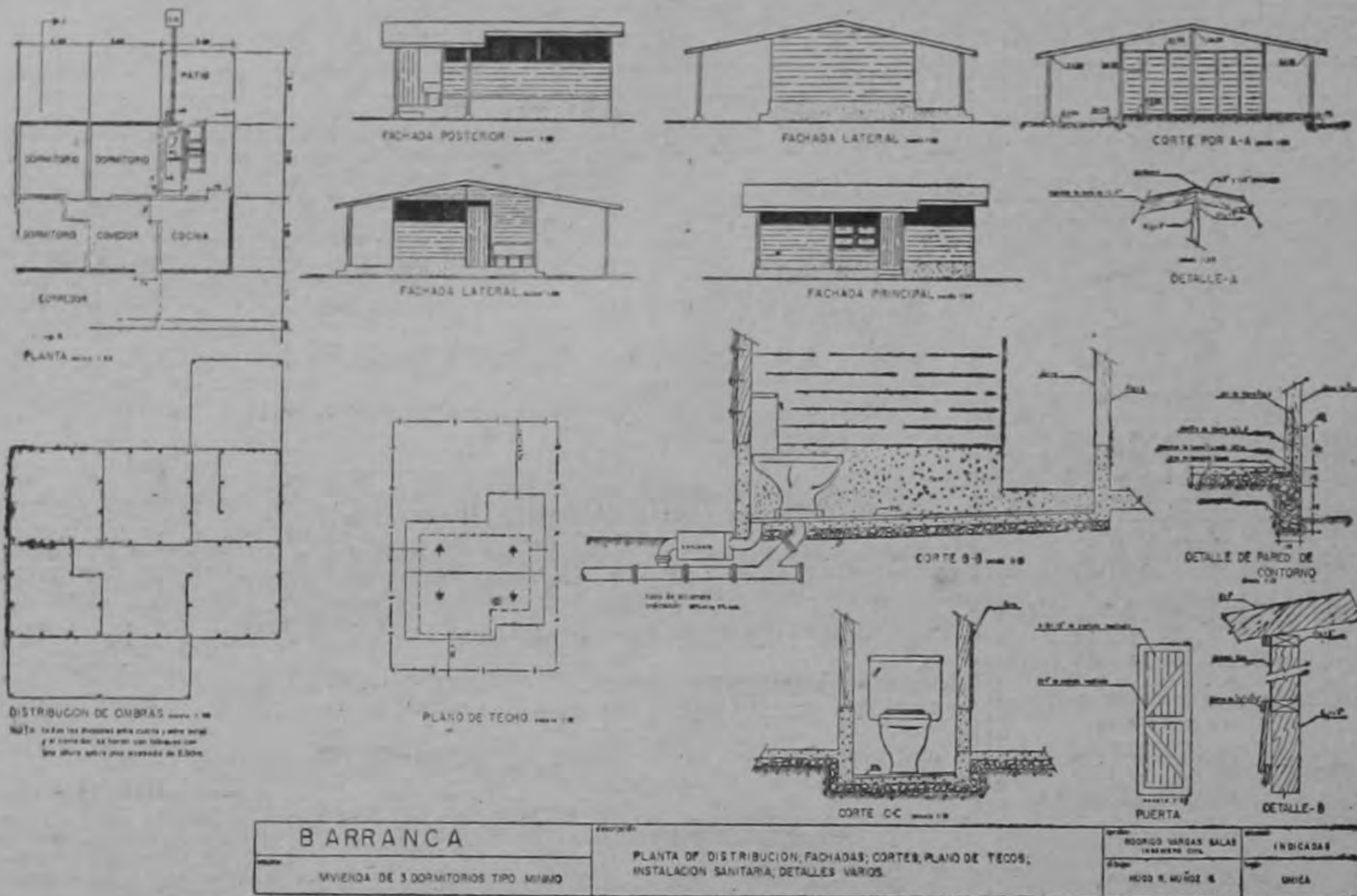
Plano del tipo de vivienda cuyo Programa inició el Instituto Nacional de Vivienda y Urbanismo en Barranca. Este programa viene a solucionar urgentes problemas de vivienda y urbanismo de aquella población, producidos por la vecindad de del río Barranca.
